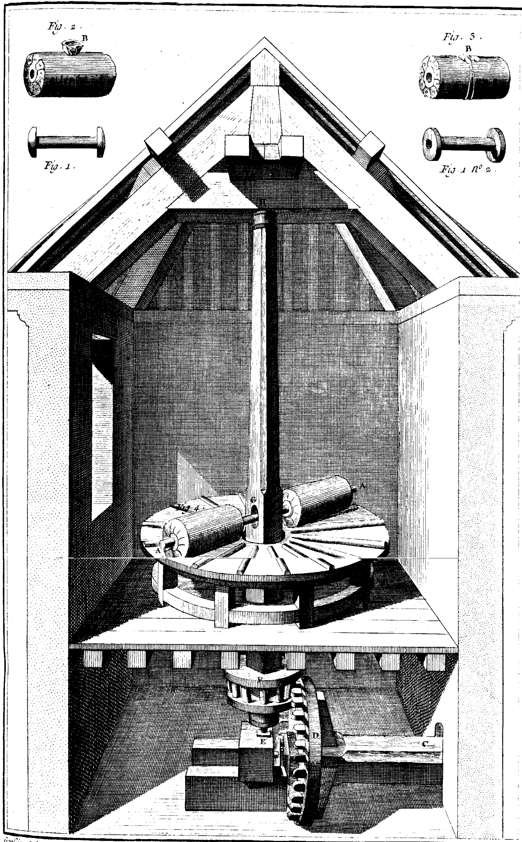
Minéralogie, Fabrique de la Poudre à Canon. Machine pour arrondir la Poudre.
