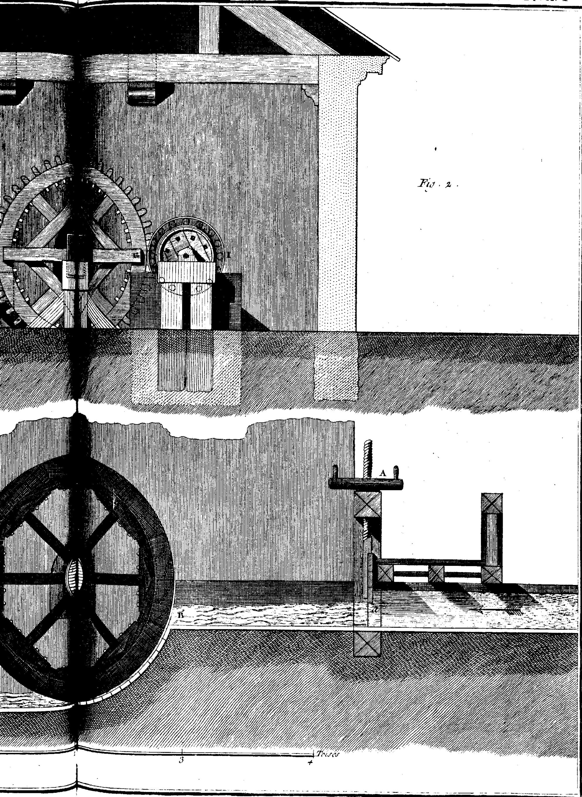
Élévation du Lijboir et Profil du Courrier de la Roue.
