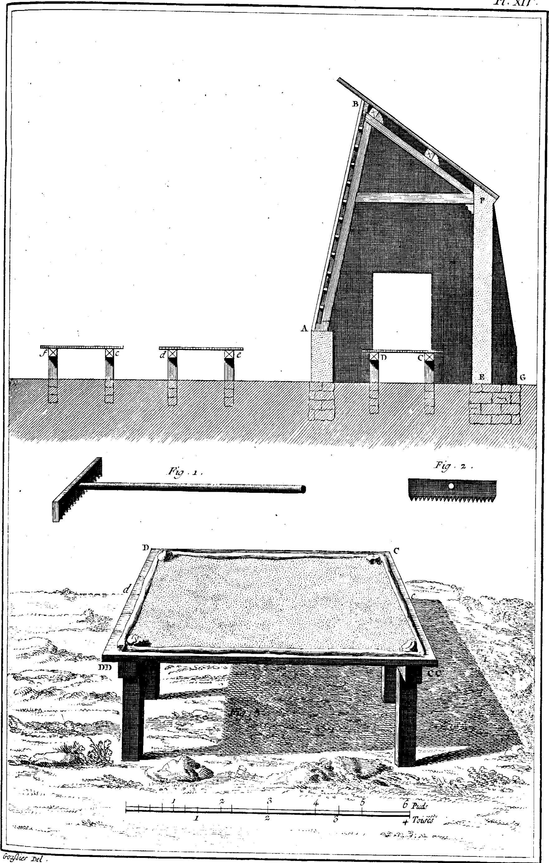
Minéralogie, Fabrique de la Poudre à Canon. Profil de l'Essorage et développements du Sechoir.
