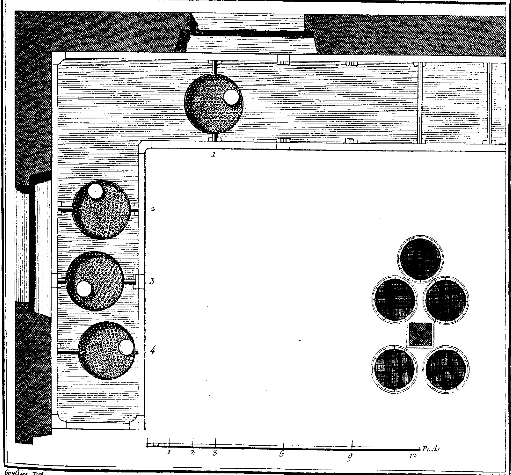
Minéralogie, l'opération de Grainer la Poudre et Plan d'un quart du Grainoir.
