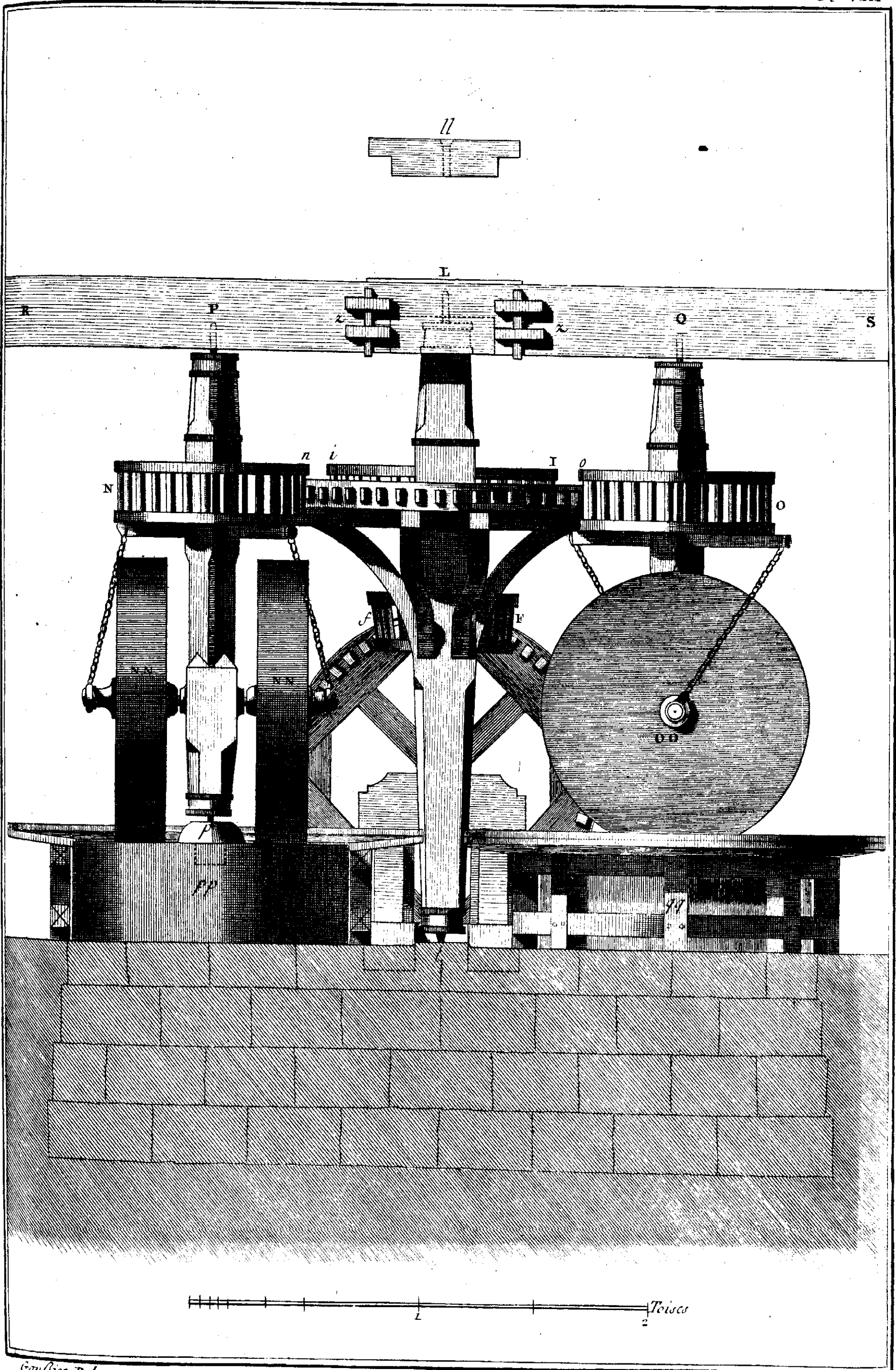
Minéralogie, Fabrique de la Poudre à Canon. Élévation transversale du Moulin à Meules roulantes.
