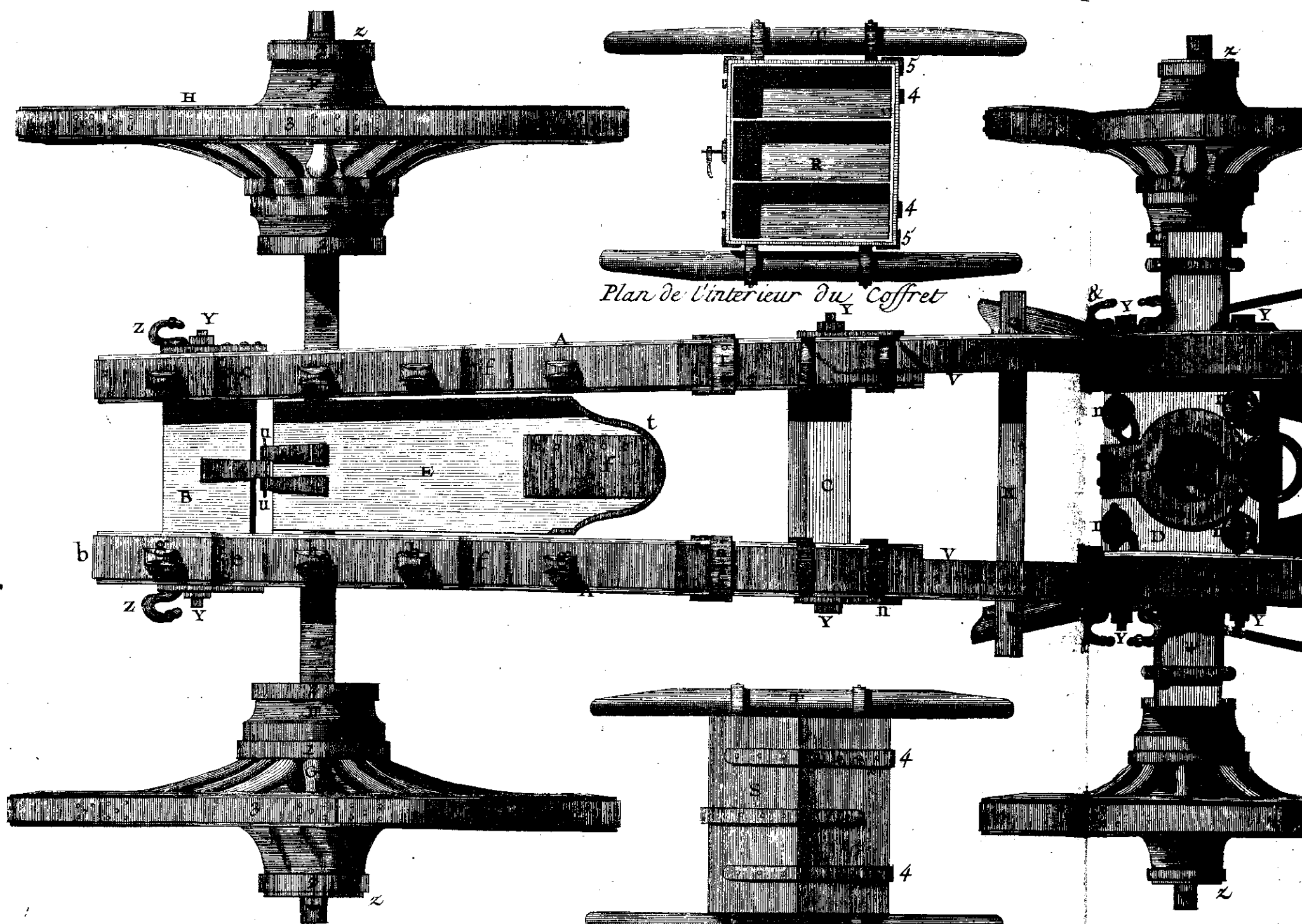
Plan du dessus du Coffret
